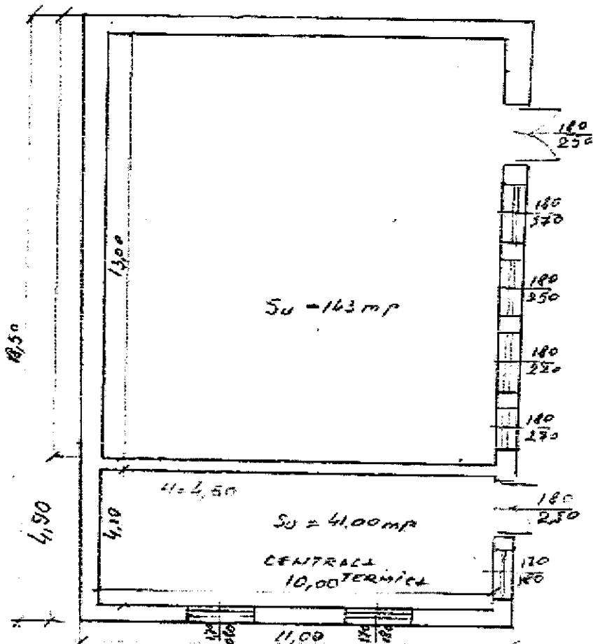
PLAN CENTRALĂ TERMICĂ
