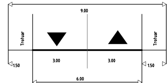
Porfil propus - strada categoria III.1 - STR. PRIMAVERII
