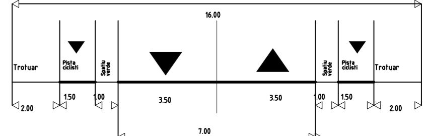
Porfil propus - strada categoria III.6b - STR. 1 DECEMBRIE 1918
