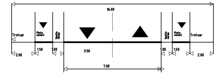
Porfil propus - strada categoria III.6b - STR. GENERAL MAGHERU Conf. PUG Caracal
