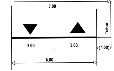
Porfil propus - strada (DRUM ACCES LOTURI) categoria III.1 conf. PUG Caracal
