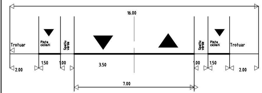
Profil propus - strada categoria III.6b - STR. GENERAL MAGHERU
