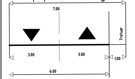
Profil propus - strada categoria III.1
