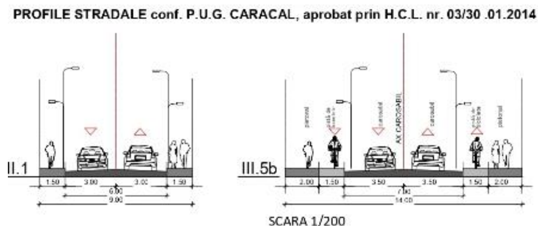
Fig. 5 Extras din Plan de reglementări PUG - profil transversal III.5b conform PUG mun. Caracal pentru strada Târgul Nou.
