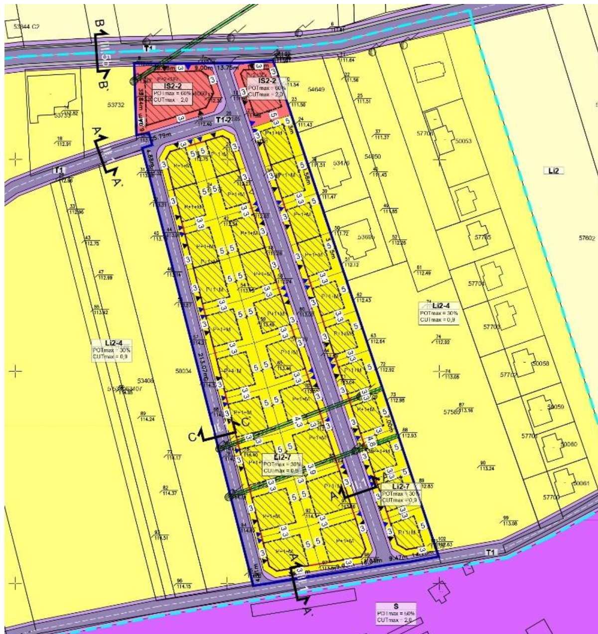
Fig. 4 Plan de situație propunere propus prin PUZ
