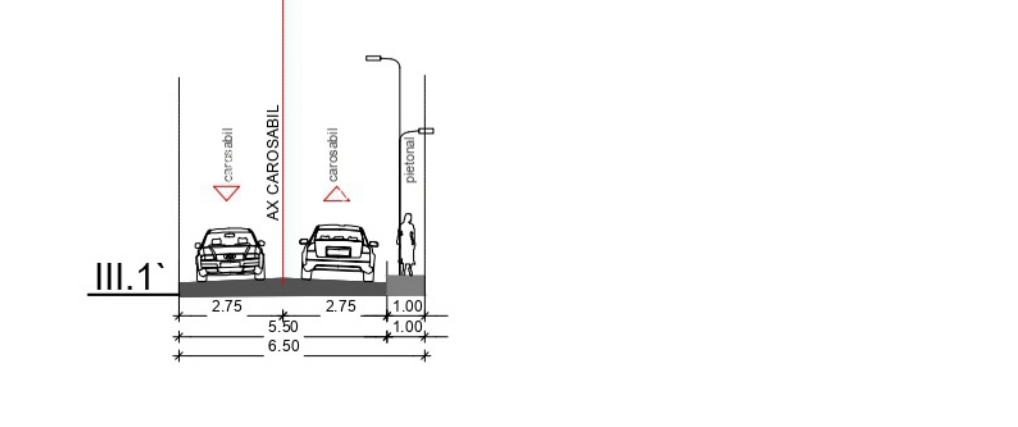
PROFIL STRADAL propus
