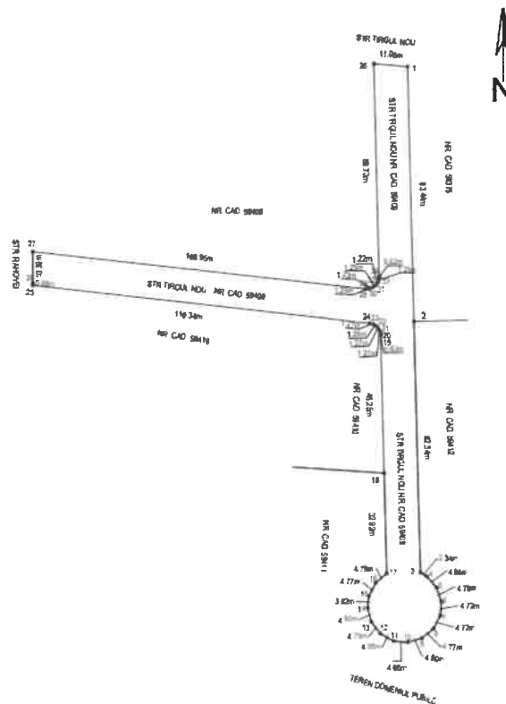
PLAN DE AMPLASAMENT SI DELIMITARE A SECTORULUI DE DRUM CE SUPLIMENTEAZĂ STRADA TÎRGUL NOU SCARA 1:1500
