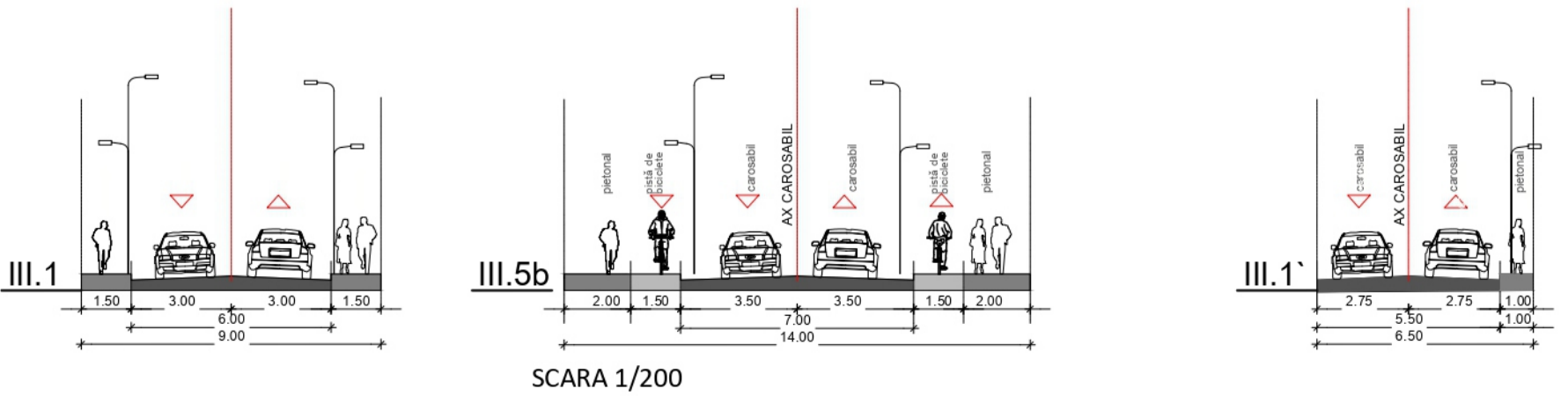
PROFILE STRADALE conf. P.U.G. CARACAL, aprobat prin H.C.L. nr. 03/30 .01.2014
