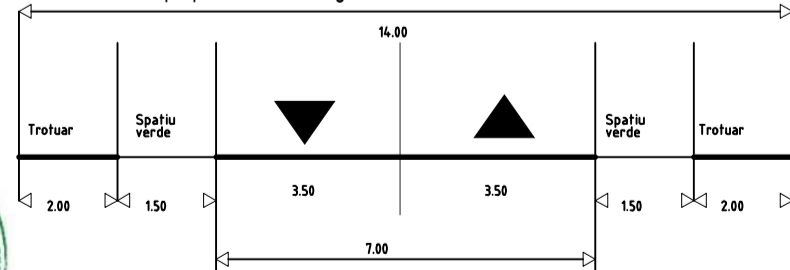
Profil propus - strada categ. III.5 - str. SALCAMULUI
