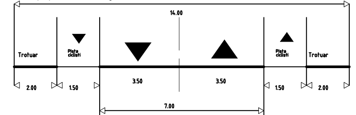
Profil propus - strada categ. III.5b - str. RAHOVEI
