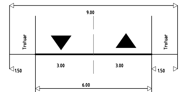
Profil propus - strada categ. III.5b - str. RAHOVEI
