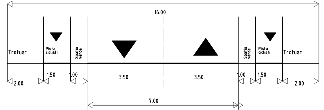
Profil propus - strada categ. III.6b - str. 1 Decembrie 1918
