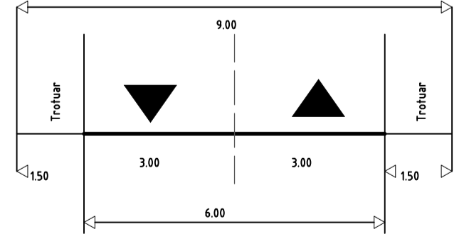
Profil propus - strada categ. III.1 - str. Primaverii
