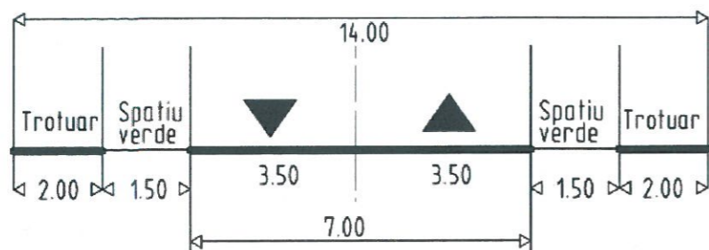
PROFIL STRADA B-DUL ANTONIUS CARACALLA
