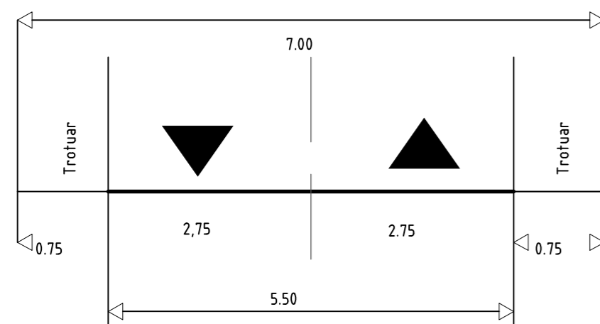
Profil propus - T1-11 (categ. III.1)
