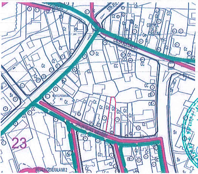
EXTRAS PUG - SITUATIE EXISTENTA - ELECTRICITATE
