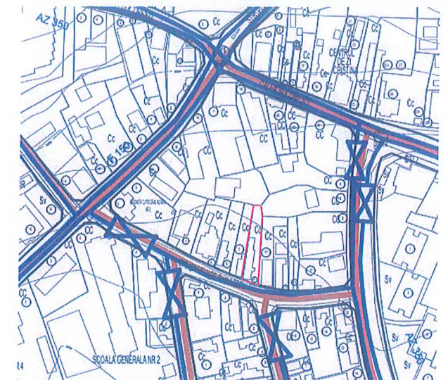
EXTRAS PUG - SITUATIE EXISTENTA - GAZE NATURALE
