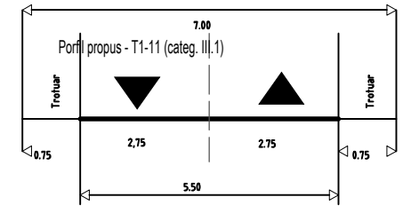
Profil propus - strada categ. III.6b - str. 1 Decembrie 1918
