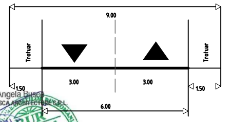
Profil propus - strada categ. III.1 - str. Primaverii
