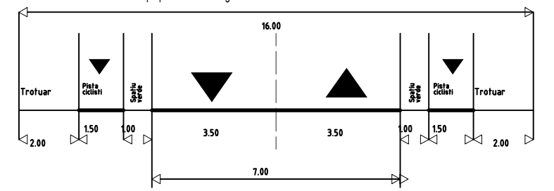
Profil propus - strada categ. III.1 - str. Primaverii
