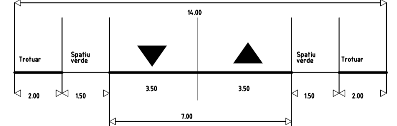
Profil propus - strada categ. III.5 - str. SALCAMULUI
