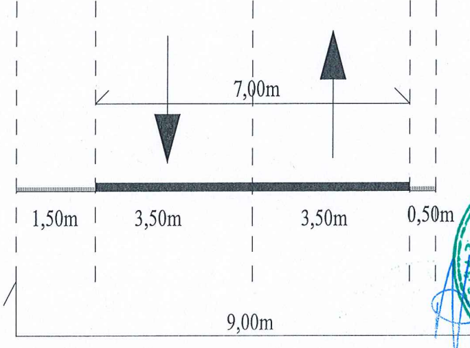
Profil stradal C-C
